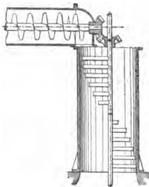
Fig. 41. — Malaxeur.
